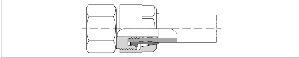
GIII.35 Compression joint, example: d16 to d20
